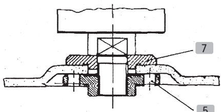
3 Poloha příruby při použití zalomených rozbíjevacích kotoučů
