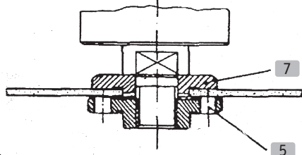
3 Position de la bride lors de l'utilisation de meules à tronçonner coudées
