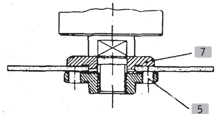
3 Položaj prirubnice kod primjene upuštenih reznih ploča
