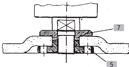
2 Poloha příruby při použití rovných rozbíjevacích kotoučů
