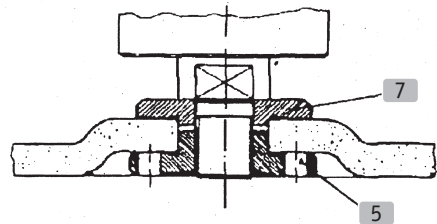
2 Položaj prirubnice kod primjene ravnih reznih ploča
