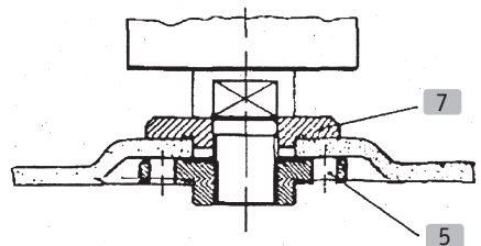
3 Položaj prirubnice kod primjene upuštenih reznih ploča
