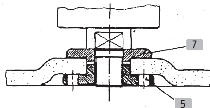
2 Flanschstellung bei Verwendung von geraden Trennscheiben
